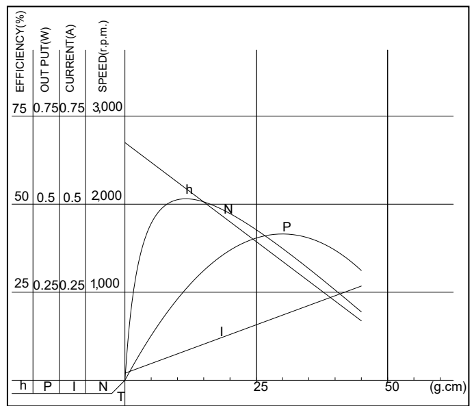
RE500CP-12560-33 6.0 V
